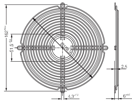
LZ37 Lüfterbaugröße 172 x 51
