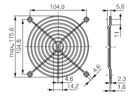
LZ30-3 Lüfterbaugröße 119 x 119
