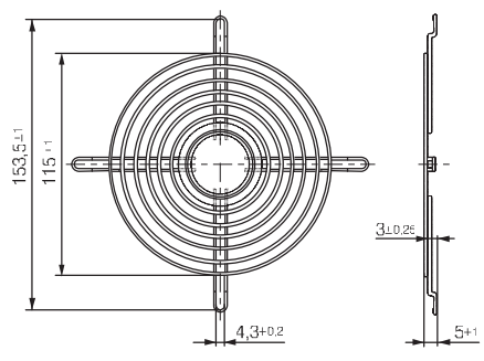
LZ30 Lüfterbaugröße 119 x 119
