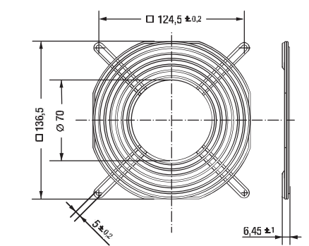
LZ53 Lüfterbaugröße 140 x 140
