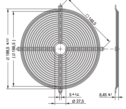
LZ22 Fan size 200 x 51
