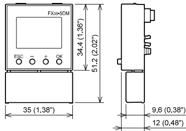
FX3S-5DM
