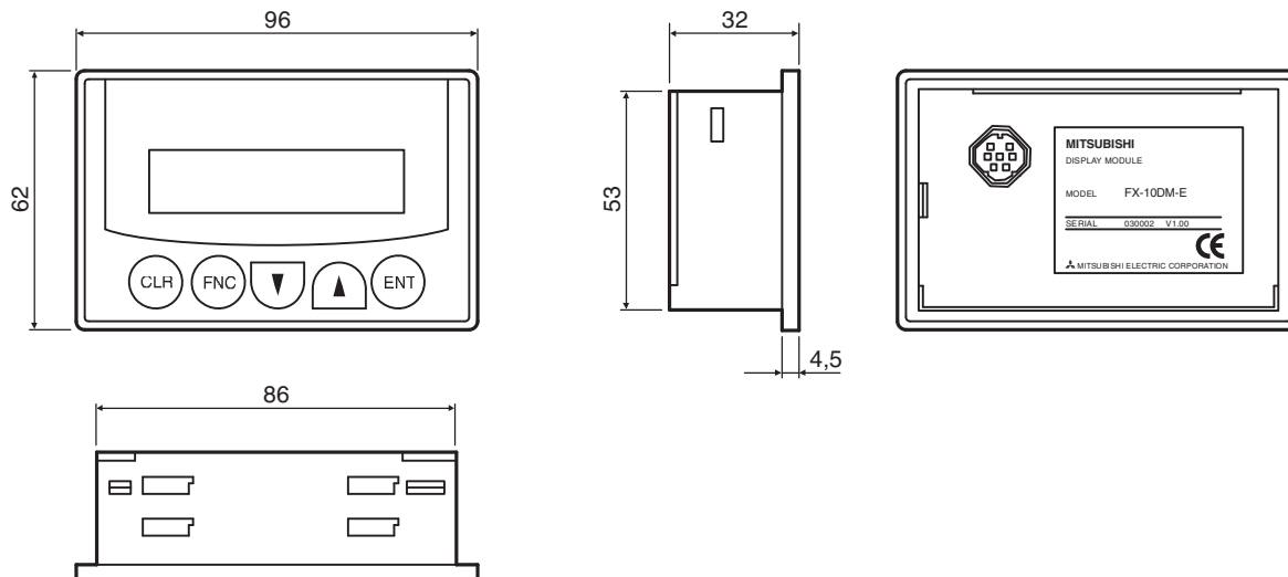
FX-10DM-E
