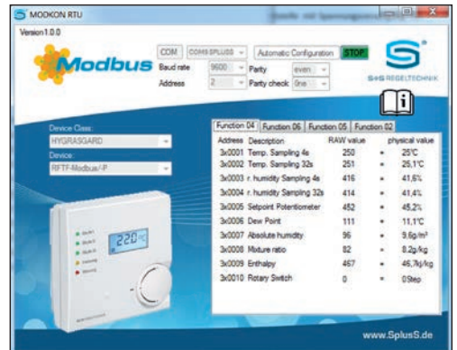
Рисунок 2 | Пример HYGRASGARD® RFTF-Modbus
