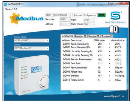
Fig. 2 | Exemple HYGRASGARD® RFTF-Modbus
