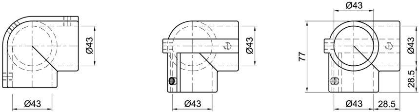
Eck-Verbinder 90°, Kopfstück, 1-schalig Corner connector 90°, Headpiece, 1-shell
